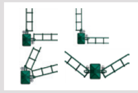
avec système de fixation colliers avec vis à métaux à tête bombée à collet carré et écrous autocassants
